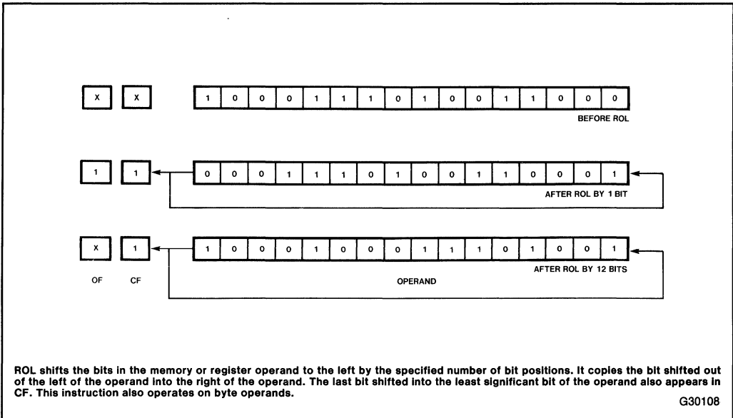
Figure 3-9. ROL
